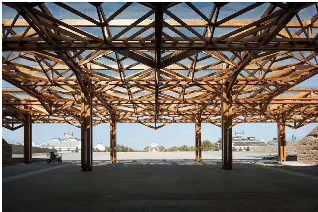
大规格耐候性竹质重组结构材在昭君博物馆的应用
