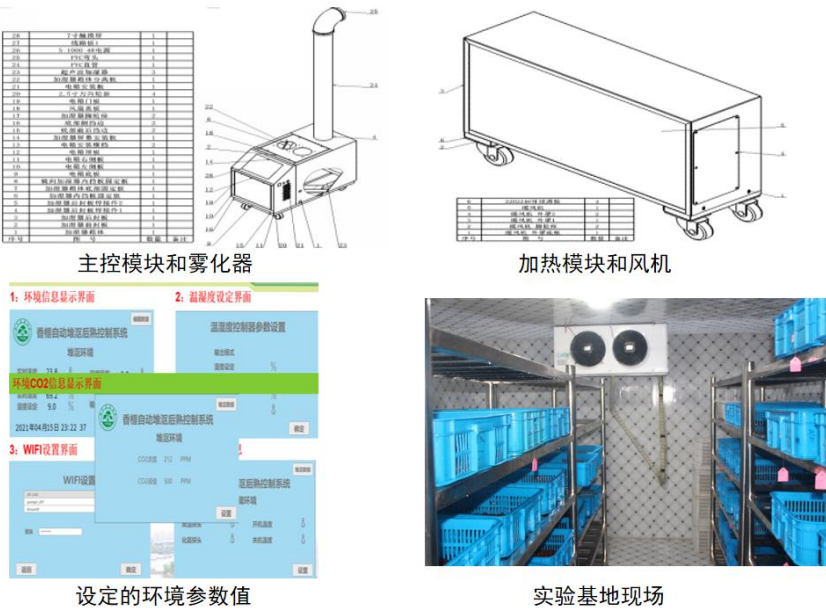
基于物联网的香榧坚果后熟智能控制装备
