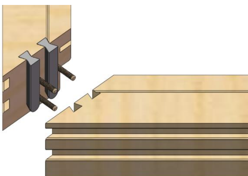
木窗角部设计构造
